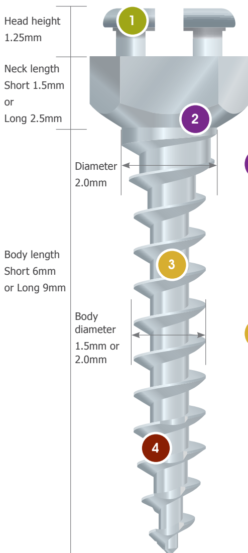
(Image shown 1.5mm Ø 9mm short neck Infinitas mini implant)
